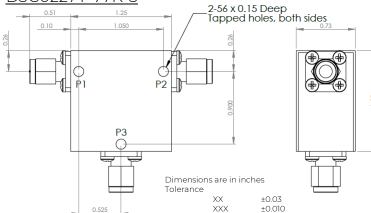
D3C0227Y-77K-3
